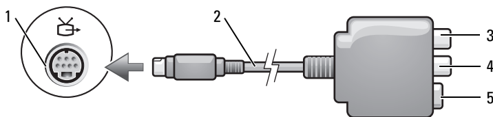
1 wyjście sygnału telewizyjnego S-video 2 adapter do przesyłania zespolonego sygnału wizyjnego 3 złącze wyjścia cyfrowego audio S/PDIF* 4 złącze wyjścia Composite Video (zespolony sygnał wizyjny) 5 złącze S-Video
