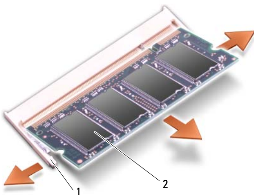
1 spinacze zabezpieczające (2) 2 moduł pamięci
